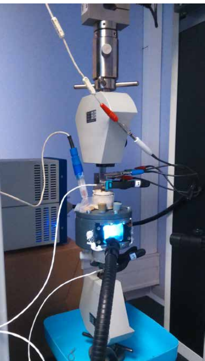
► Couplage émission acoustique et bruit électrochimique dans le suivi des phénomènes de corrosion sous contrainte
