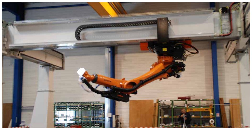
► Portique équipé de 2 robots (14 axes pilotés) dotés de changeurs d'outils adaptés aux différentes technologies CND envisagées pour le contrôle de l'intégrité des conteneurs métalliques de déchets radioactifs - Installation de type Lucas/Clemessy
